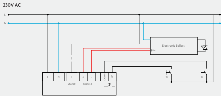
DD-VERSION (DALI/DSI)
