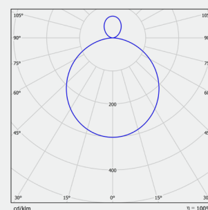
KVILL PE OP
