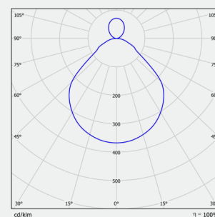
KVILL PE MP
