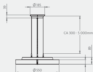
KVILL PE Ø550 mm OP/MP
