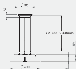
KVILL PE Ø400 mm OP/MP
