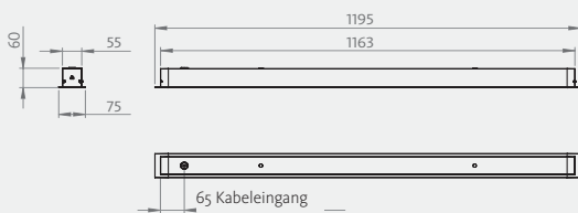
SEVEDE 1200 mm
