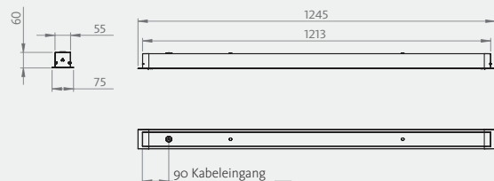
SEVEDE 1250 mm
