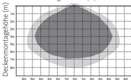
Deckenmontagemuster (m)
