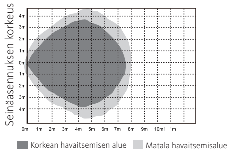
Seinäasennuksen kuvio(m)
