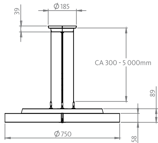
Kvill PE 750
