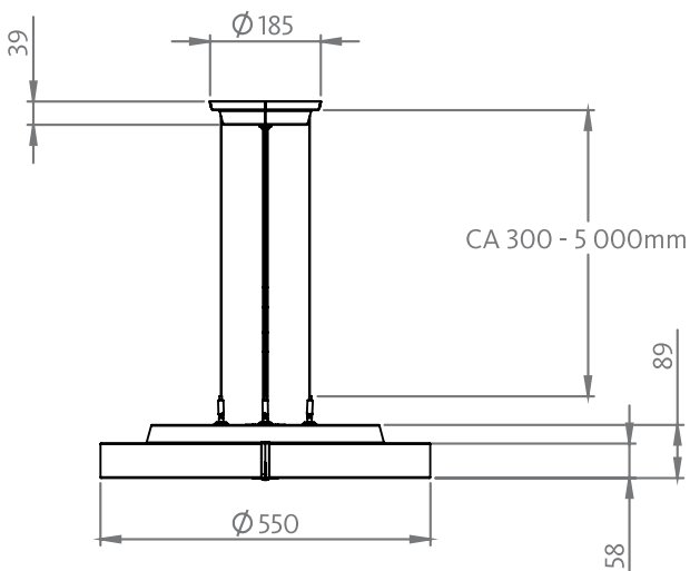
Kvill PE 550
