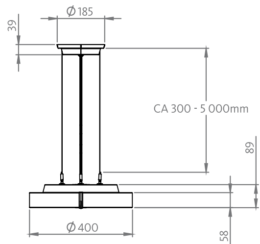
Kvill PE 400
