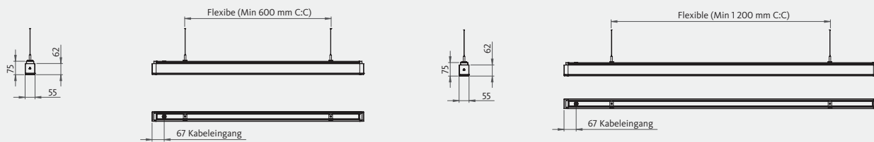
SEVEDE PE 1200 mm
