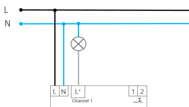
PRM-AUSFÜHRUNG – AUTOMATIK-MODUS
