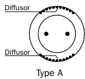
Diffusor-segment: 2x80° SIGNETTE D
